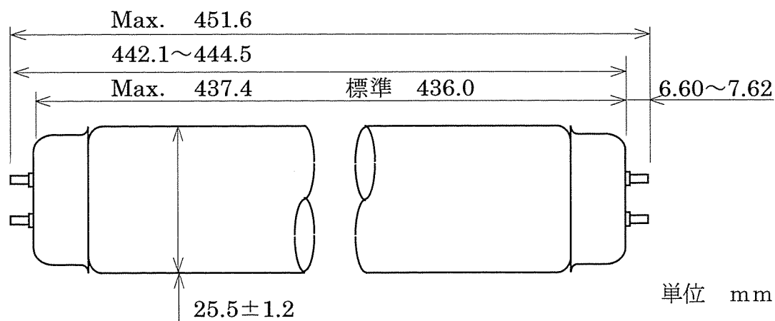
白色蛍光ランプ（直管形） 〈サンライン〉
